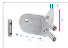
Pfostenhalter ca. 50mm Wandabstand, Außenecke Support pour poteau distance du mur 50mm angle extérieur
